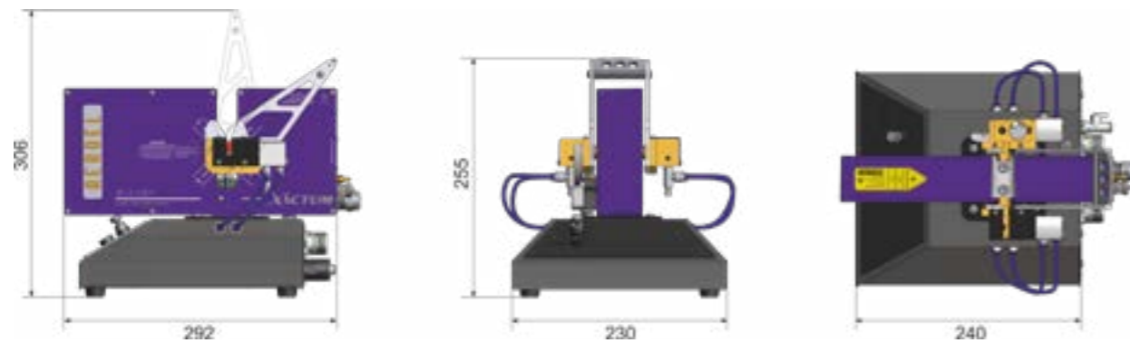
寸法はすべて mm 単位。ケーブルとコネクタなしの寸法。
