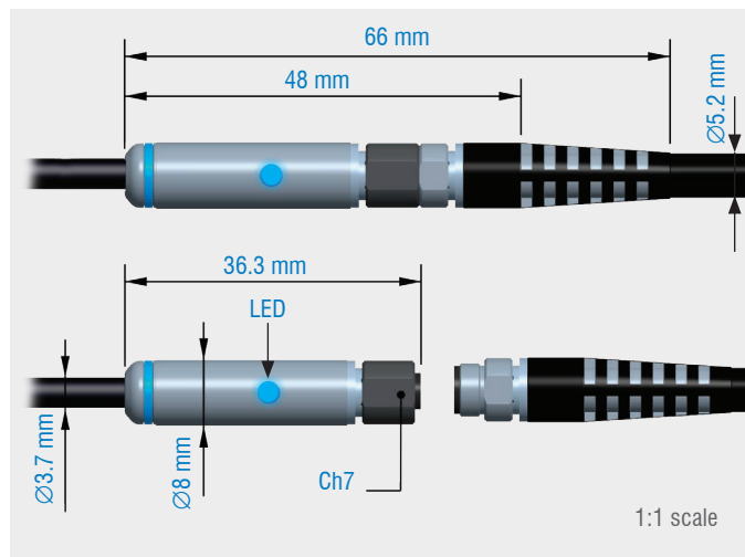
Dimensión conector SMART
